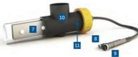
Ogniwo elektrolityczne
